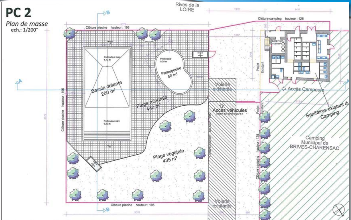
Plan de la future piscine au camping d'Audinet.
